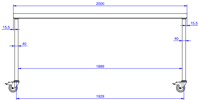
Front aanzicht
